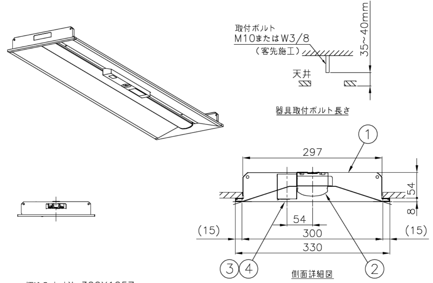
埋込み穴寸法 300X1257
