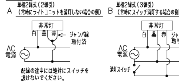
配線図
