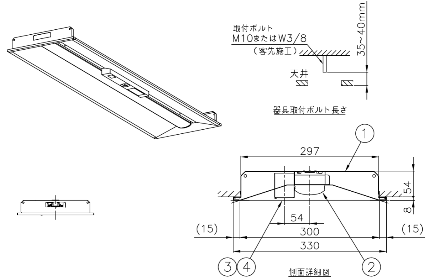
埋込み穴寸法 300X1257
