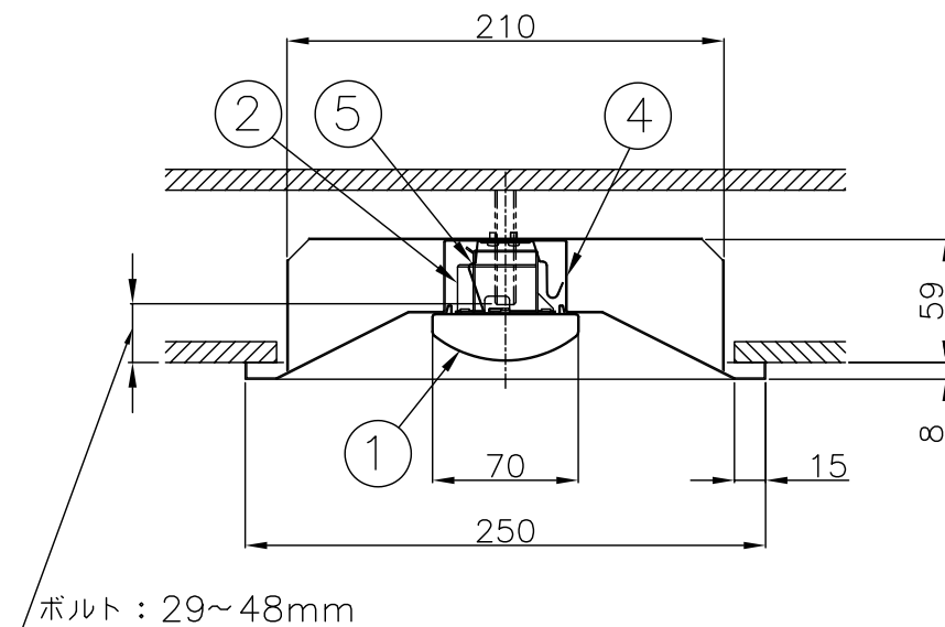
埋込み穴寸法 220×617(単体)
