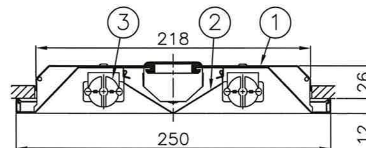
断面詳細図 (1/3)
