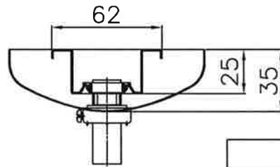
断面詳細図1/3
