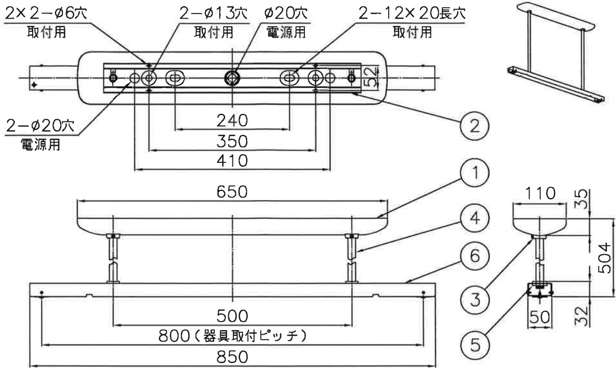
断面詳細図1/3
